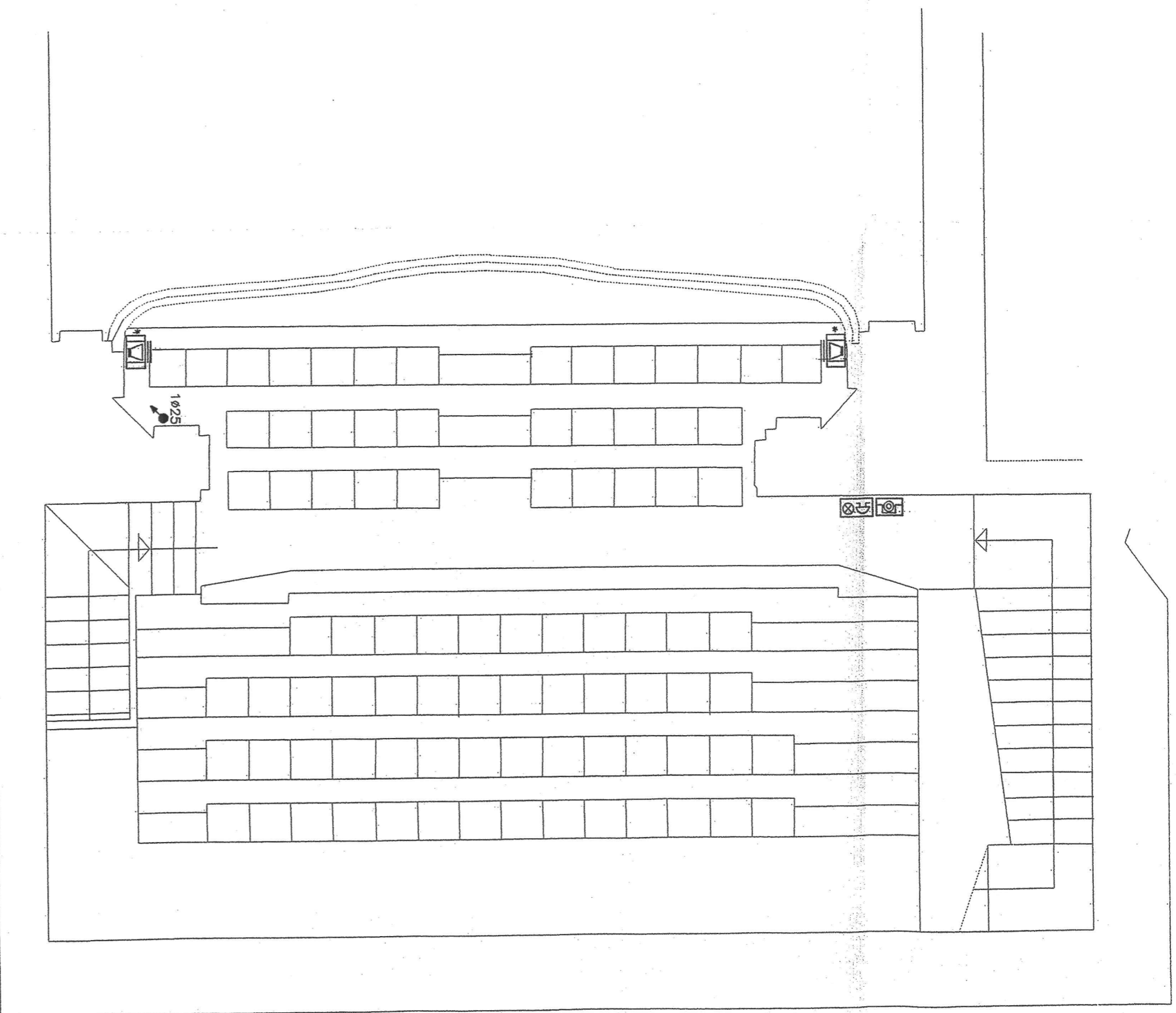
PIANTA A QUOTA +7.5m
