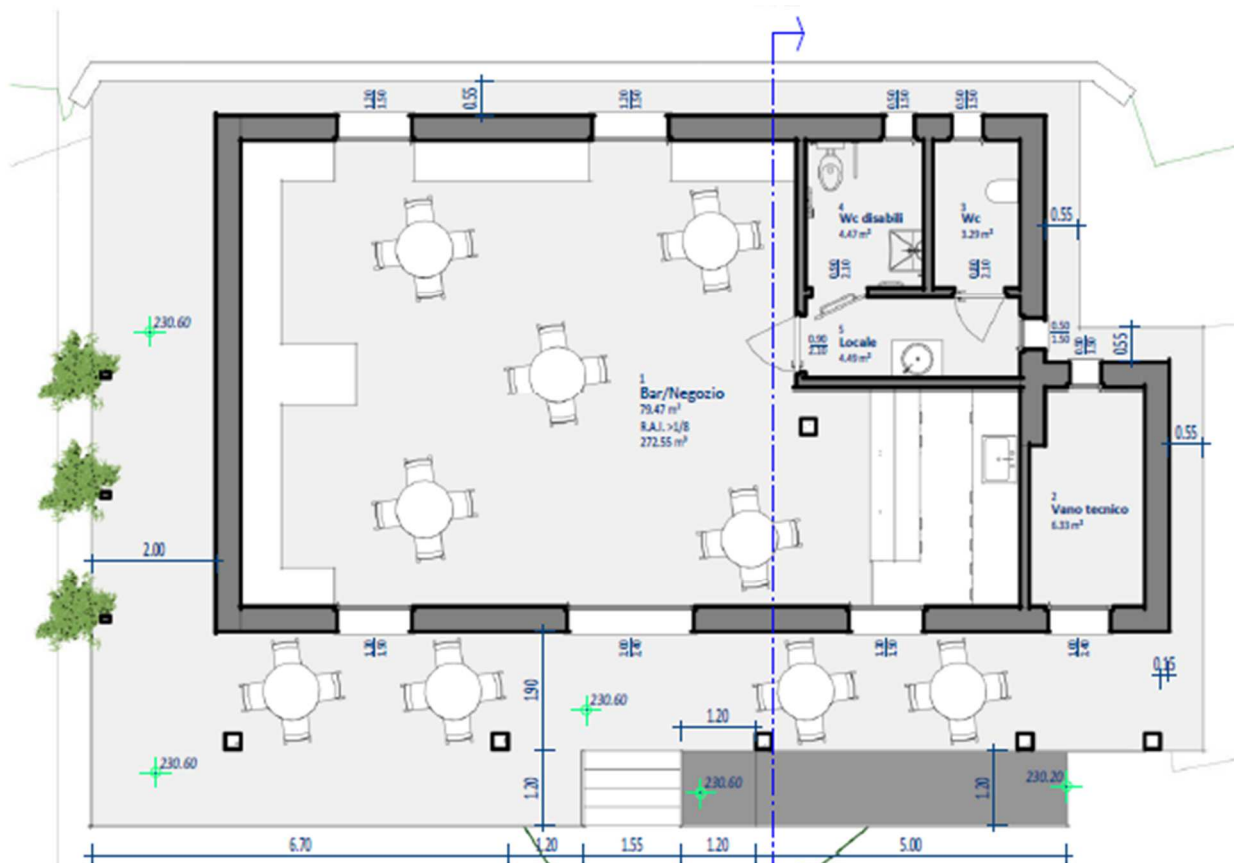
Pianta di progetto
